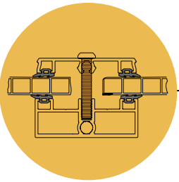
Bevestiging van twee polycarbonaat platen.
