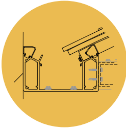
Detailtekening van profielen en montage.
