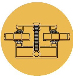
Bevestiging van twee polycarbonaat platen.
