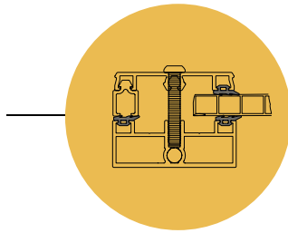
Bevestiging van polycarbonaat in een zijsluitprofiel.
